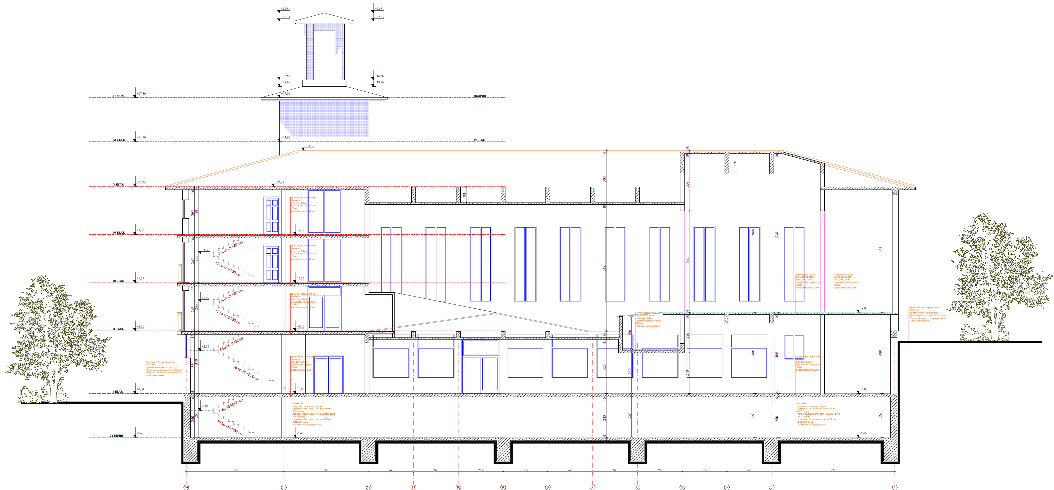
РАЗРЕЗ A-A
